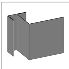
VB21 Profilé d'angle avec retour de recouvrement
