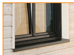
Appui sur bardage bois
