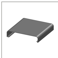
CD 09 Couvertine d'acrotère à fixation mécanique avec plis rayonnés
