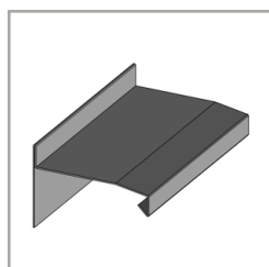
IS54 Couronnement à double pente avec arrêt et fixation verticale
