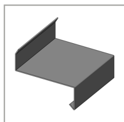
IS56 Goutte d'eau avec fond de joint
