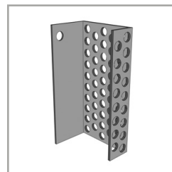
Arrêt latéral avec retour d'enduit
