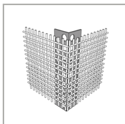
Profilé d'angle avec trame
